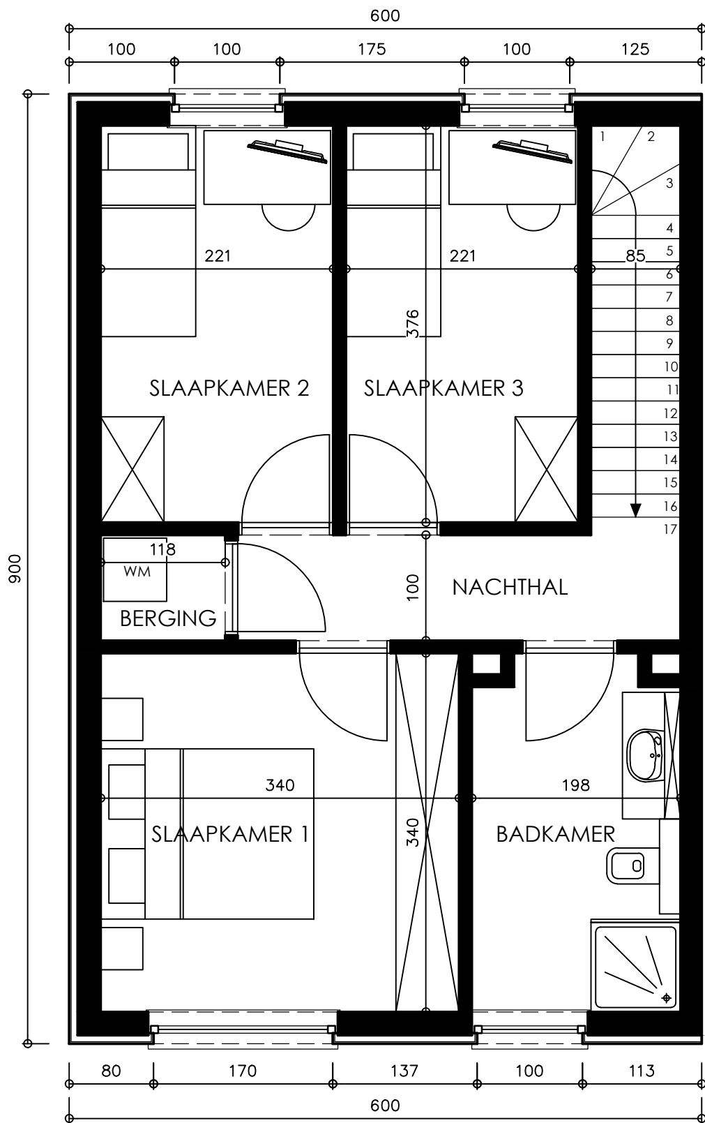
VERDIEPING 1
